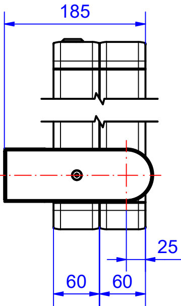
profiles 60-60
