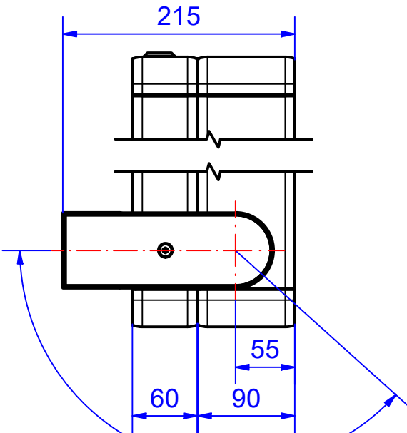
profiles 90-60
